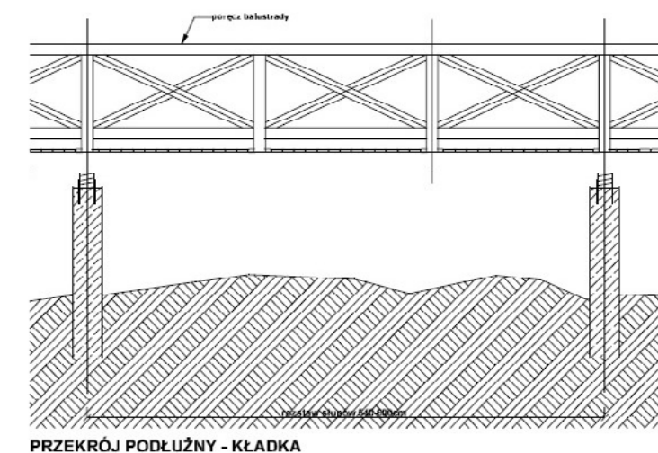
PRZEKRÓJ PODŁUŻNY - KŁADKA
